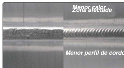
Soldadura TIG estándar (a 60A)
